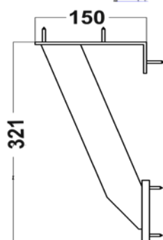
Rückwandkonsole „AKO 5“ Höhe 321 mm
