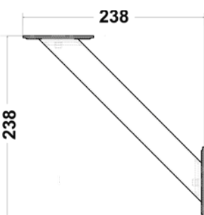
Rückwandkonsole „RWK 45“ Rohr Ø 45 mm
