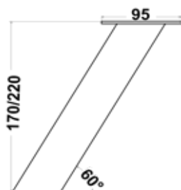
Barkonsole Ischia schräg, 170x50x50mm
