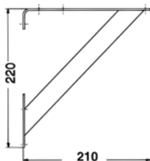
Rückwandkonsole „RAK“ Höhe 220 mm
