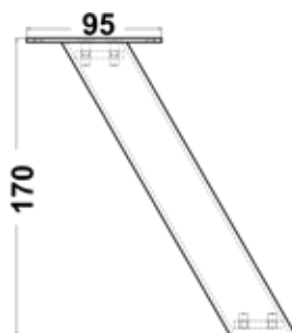
Barkonsole „BKO Light“ Höhe 170mm
