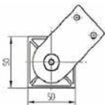
Sockelfuß Capri, 30mm höhenverstellbar, 50x50mm
